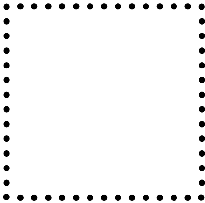
مُرَبَّع
