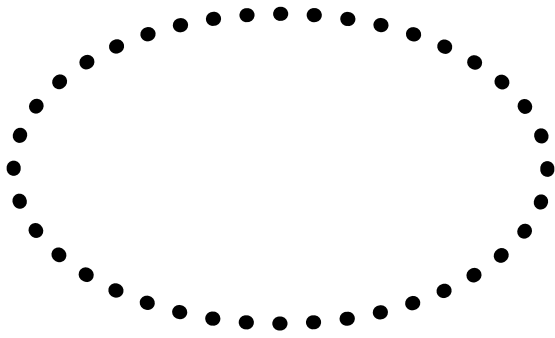
بَيْضَوِي
