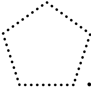
مُخَمَّس
